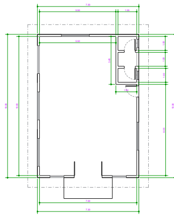
PLANTA TIPO - BARRACÃO FECHADO ESC. 1/50
