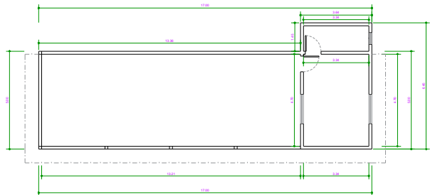
PLANTA TIPO - BARRACÃO ABERTO ESC. 1/50
