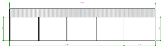
ELEVAÇÃO FRONTAL - BARRACÃO ABERTO ESC. 1/50
